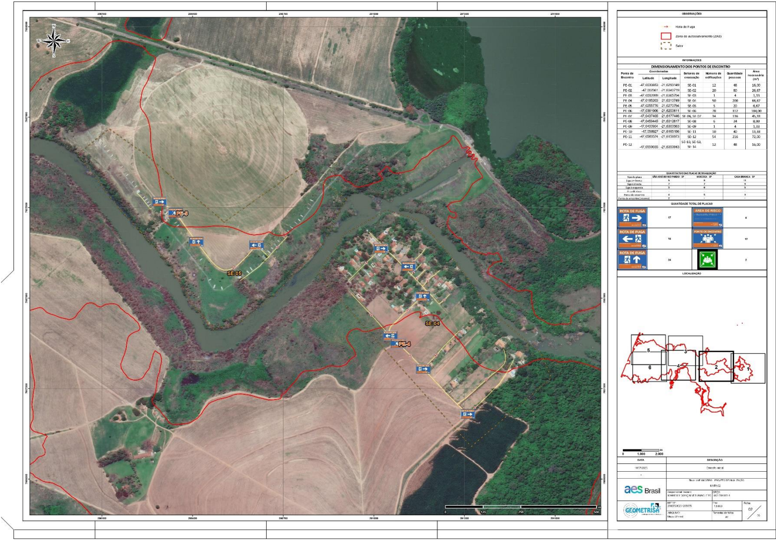
Figura 23 – Mapa de projeto de sinalização da UHE Limoeiro – Mapa 2
