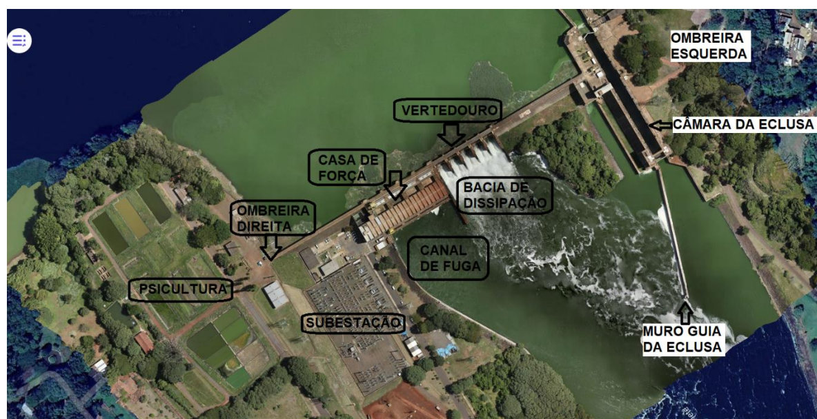
Figura 5 – Arranjo geral da barragem da UHE Barra Bonita
