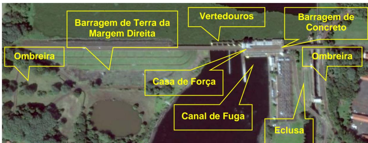
Figura 5 – Localização das Estruturas da Barragem da UHE Bariri.
