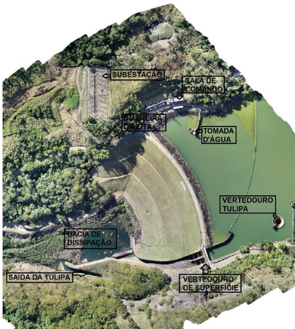
Figura 5 – Arranjo geral da barragem da UHE Euclides da Cunha
