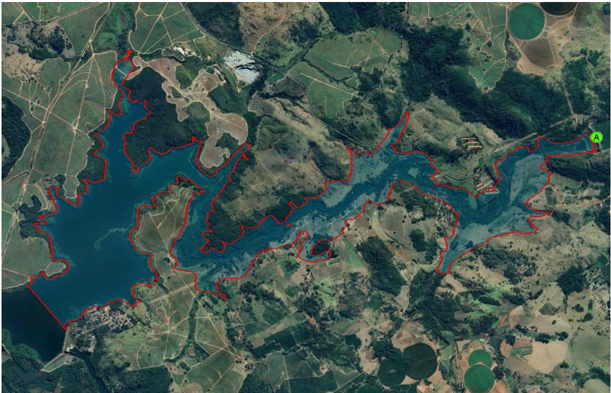
Figura 3 – Zona de Autossalvamento da UHE Euclides da Cunha
