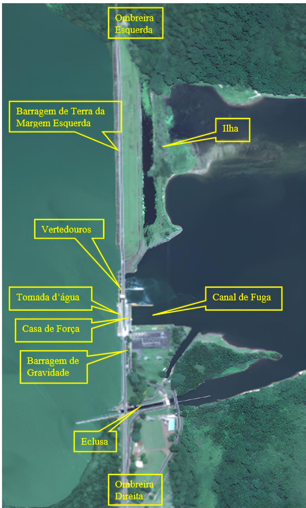
Figura 5 – Arranjo geral da barragem da UHE Ibitinga
