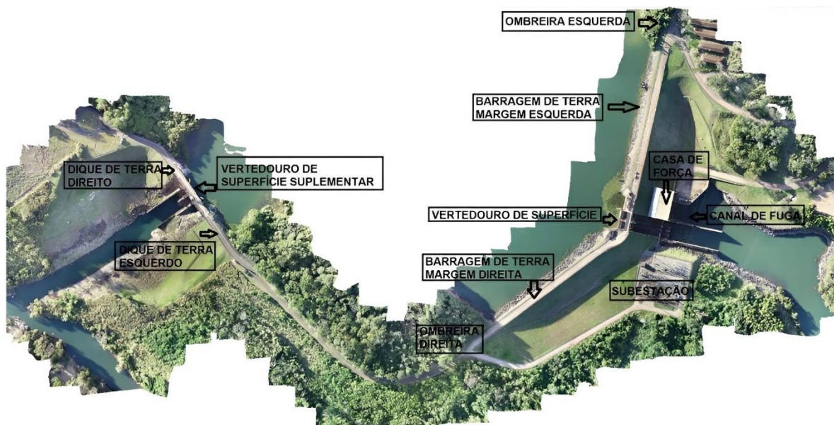
Figura 5 – Localização das Estruturas da Barragem da UHE Limoeiro.
