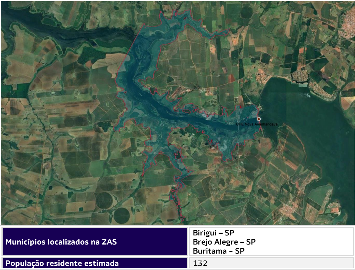
Figura 3 – Zona de Autossalvamento da UHE Nova Avanhandava
